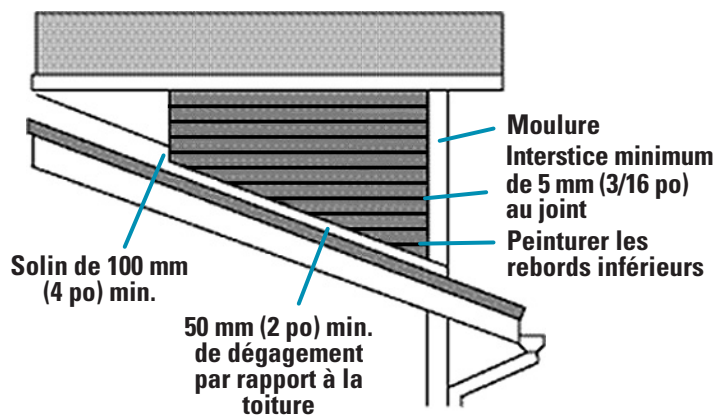
FIGURE 2 VUE DÉTAILLÉE D'UN SOLIN DE TOIT
