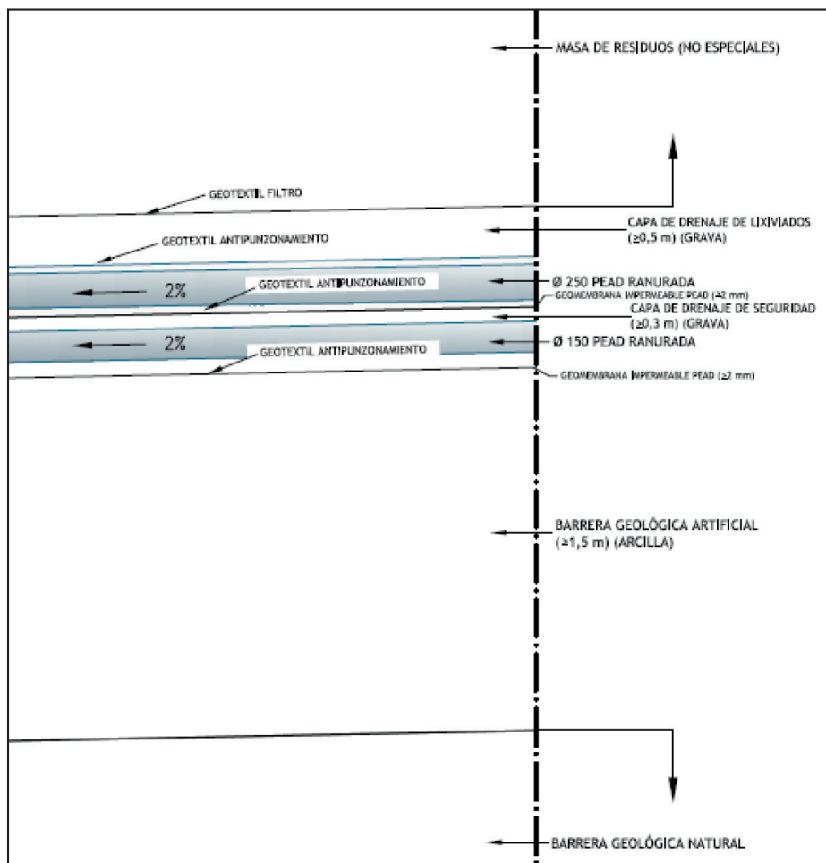
Figura 7. Sección tipo del vertedero de Flix según proyecto constructivo original (Capas de protección del sellado basal).
