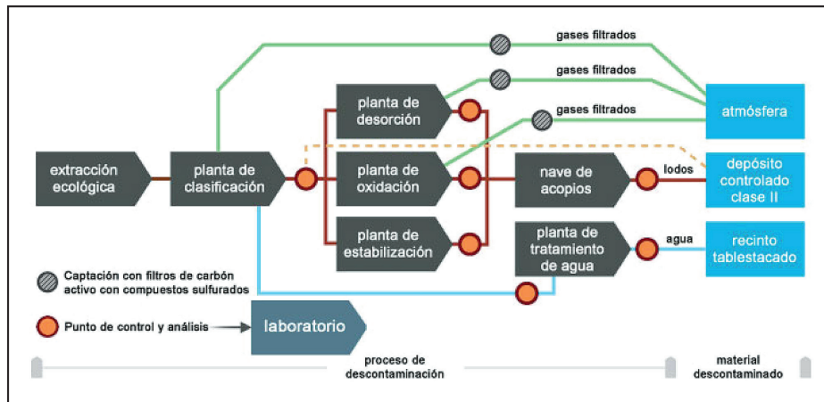
Figura 6. Proceso tratamiento lodos contaminados.
