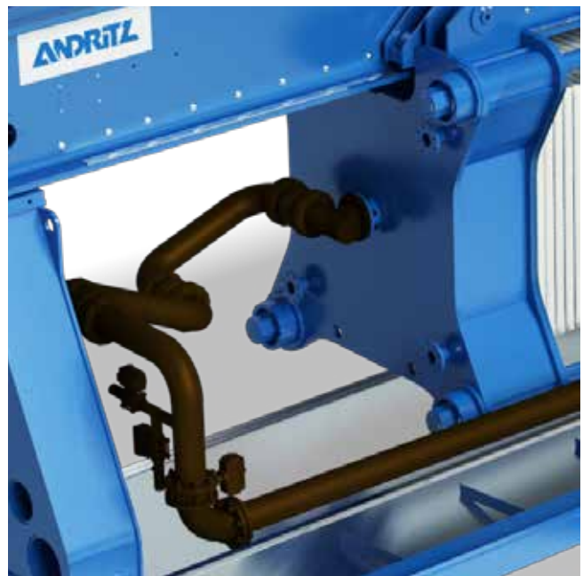
Segunda entrada de alimentación para tiempos de ciclo más cortos
