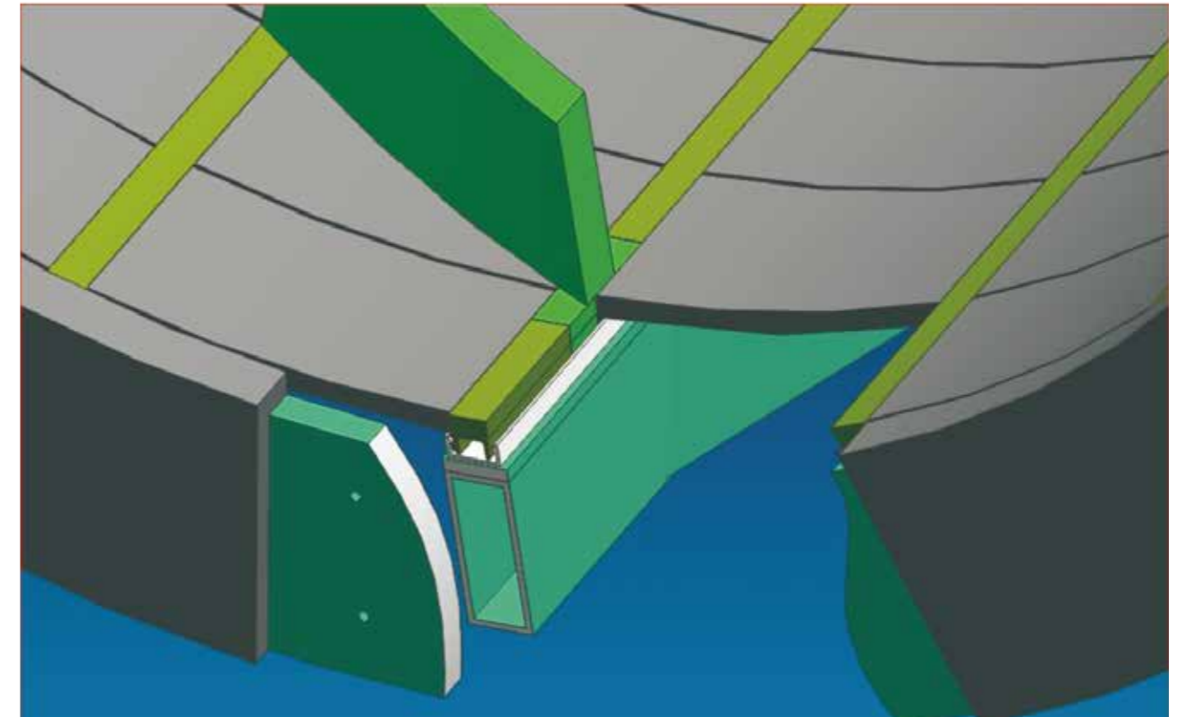
Ilustración de la instalación de Malla de Trommel
