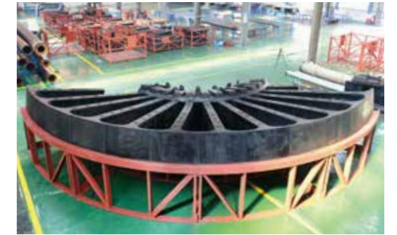
Revestimiento tapa de descarga en molino AG de \varnothing 12.2 \times 11\text{m}
