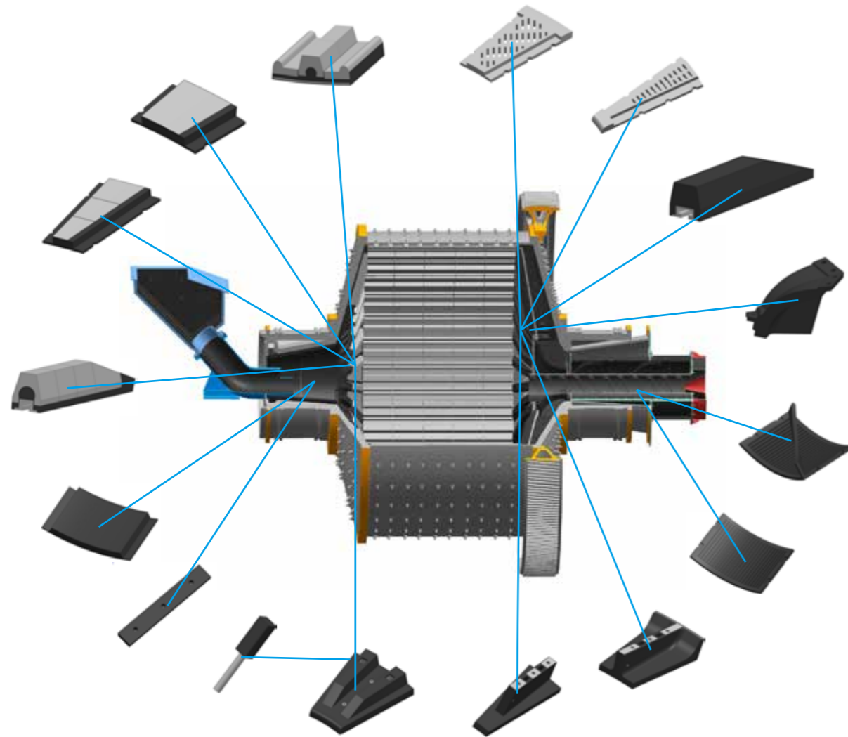
Una ilustración de distribución de piezas de repuesto de molino
