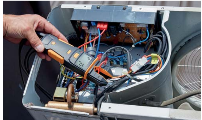
Comprobación de corriente en un compresor con testo 755 .
