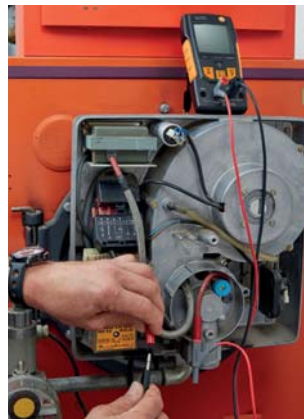
Medición de µA para comprobar la corriente de ionización.
