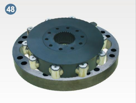
ZF:PLM-7/9 Motor
