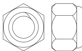
Porca de Travamento M12 (50)–1
