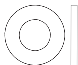
Rondelle M8 (44)–8
