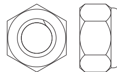
Porca de Travamento M10 (32)–4
