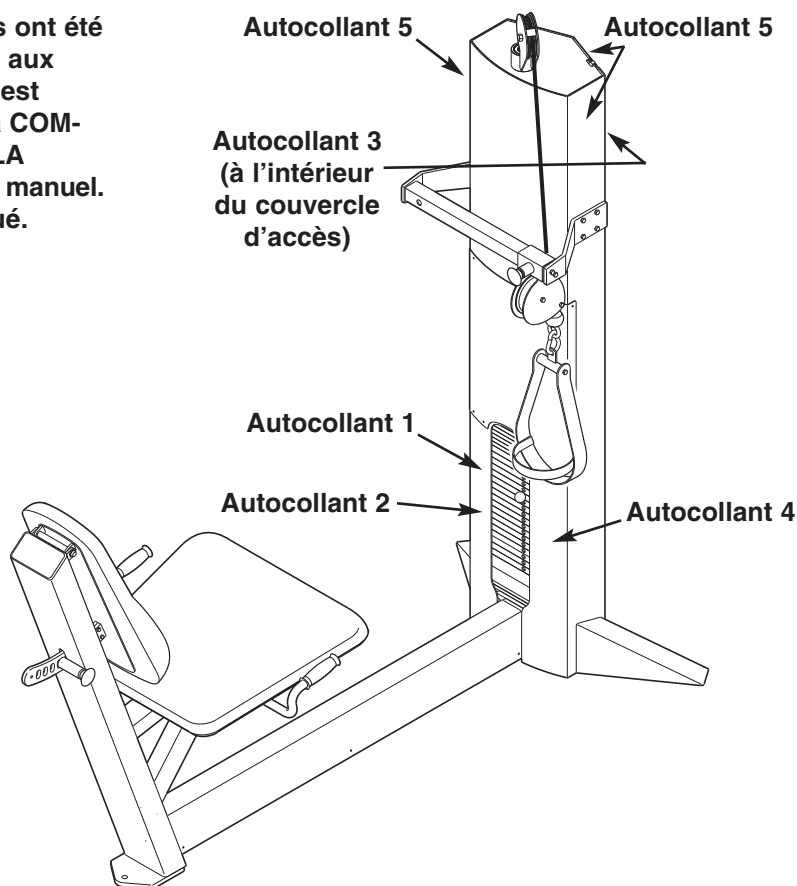
Autocollant 1 Illustré à 68% de la taille réelle Pièce GZ7003
