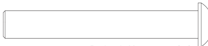
Boulon de M12 x 86mm (77)
