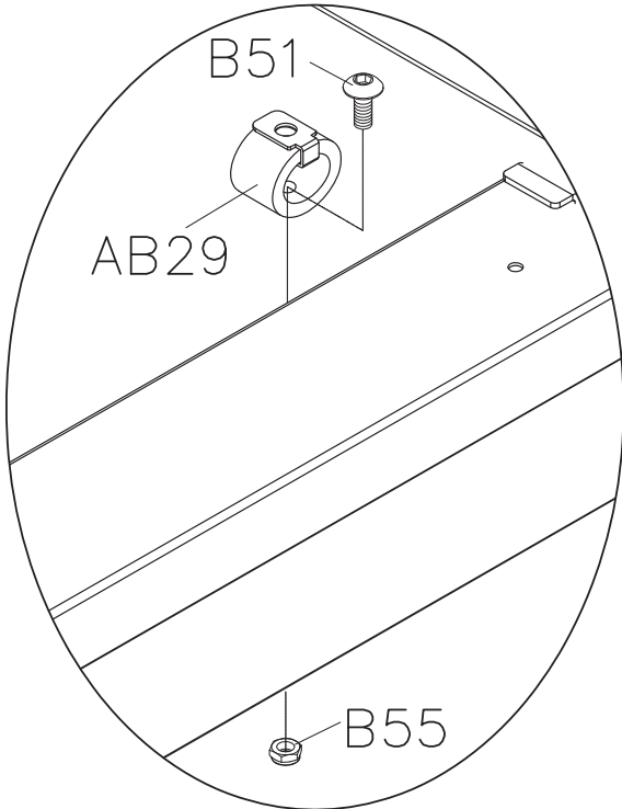
B 詳圖(1: 5)
