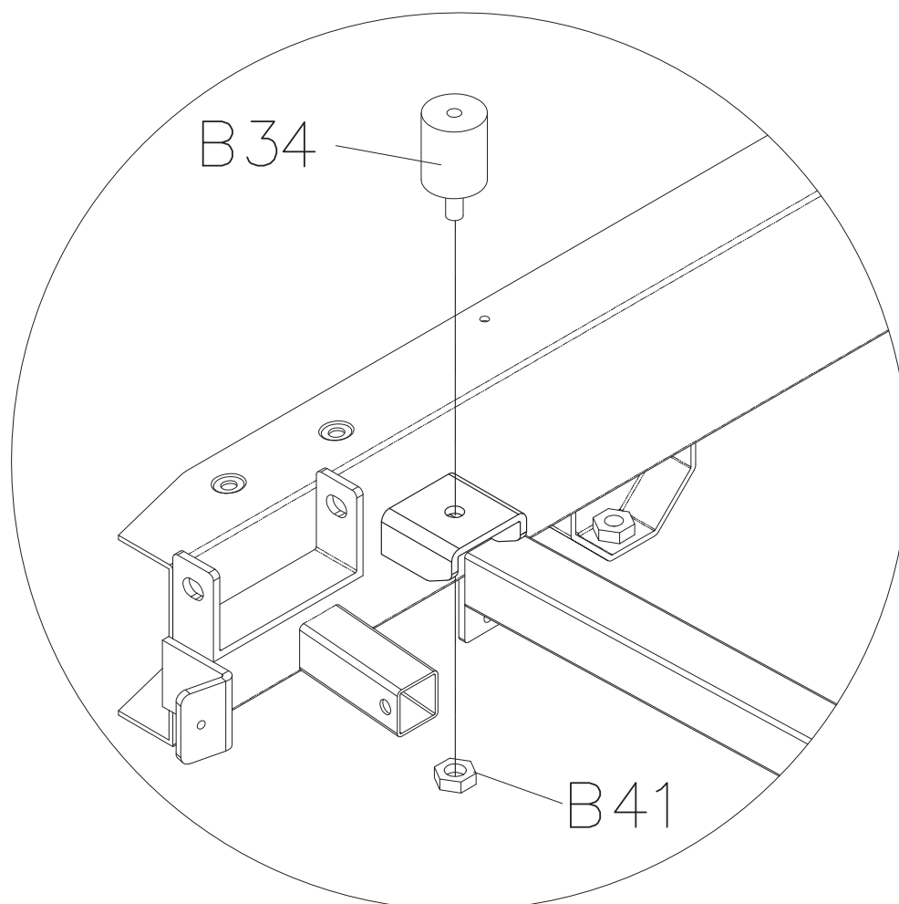
A 詳圖(1:5)
