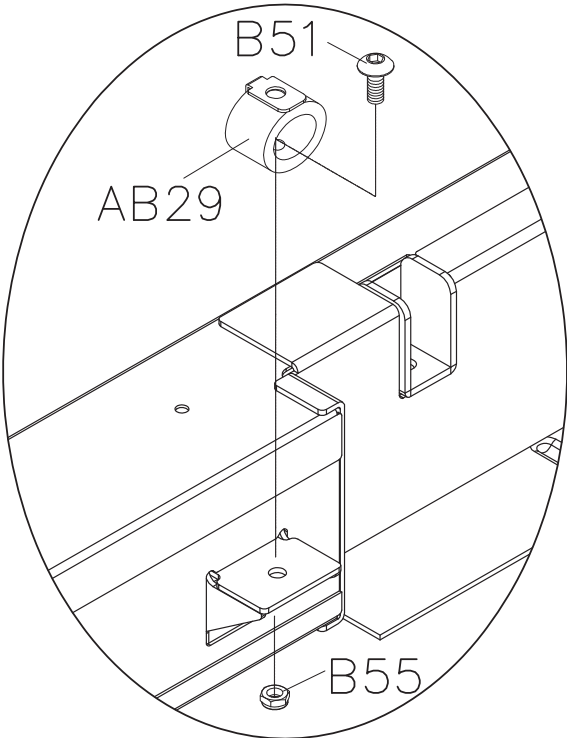
A 詳圖(1: 5)
