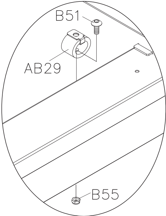
B 詳圖(1: 5)
