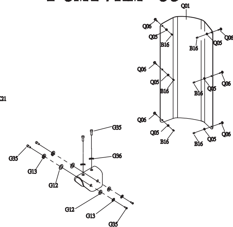
AG1拆卸連接組 詳圖
