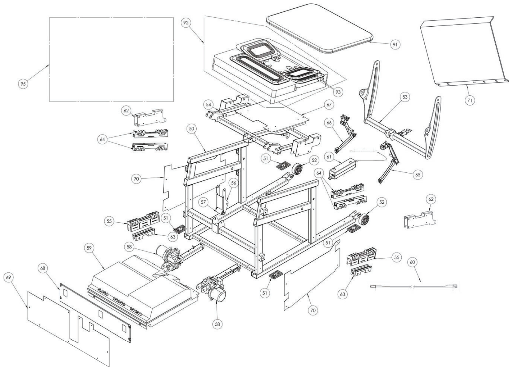
椅子下部分解图
