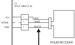
Polar Cable AK36-00021-0003
