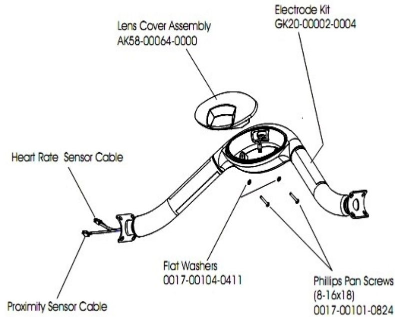
ERGO Bar Assembly – AK58-00018-0000
