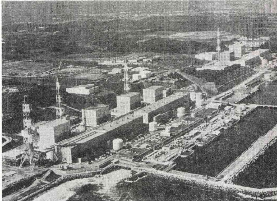
↑ 東電福島第1原子力発電所は、太平洋に臨む福島県の大熊、双葉両町にまたがる約320万平方メートルの敷地に建設された。
