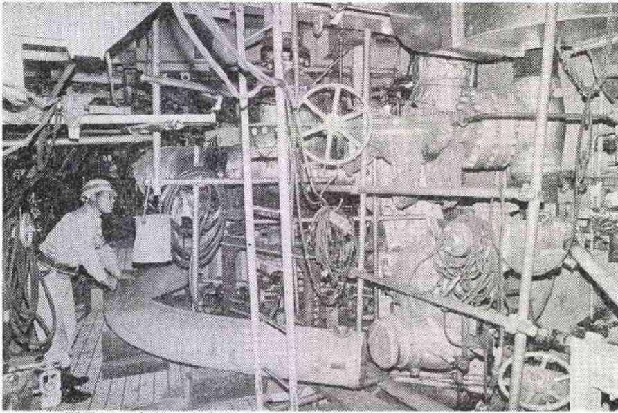
↑ 原子炉の底部。大小多くのパイプ類が入り乱れている。
