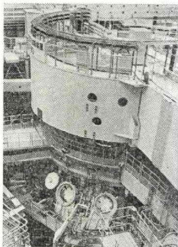
核融合実験装置JT-60の本体（茨城県那珂郡那珂町の日本原子力研究所）
