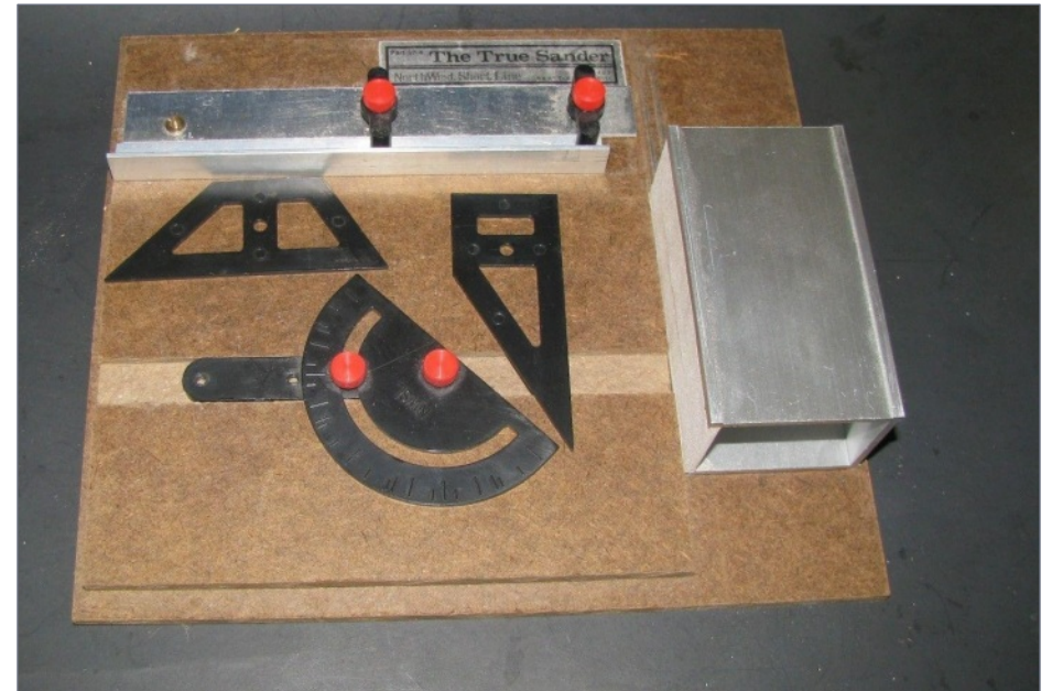
26. NWSL True Sander.
