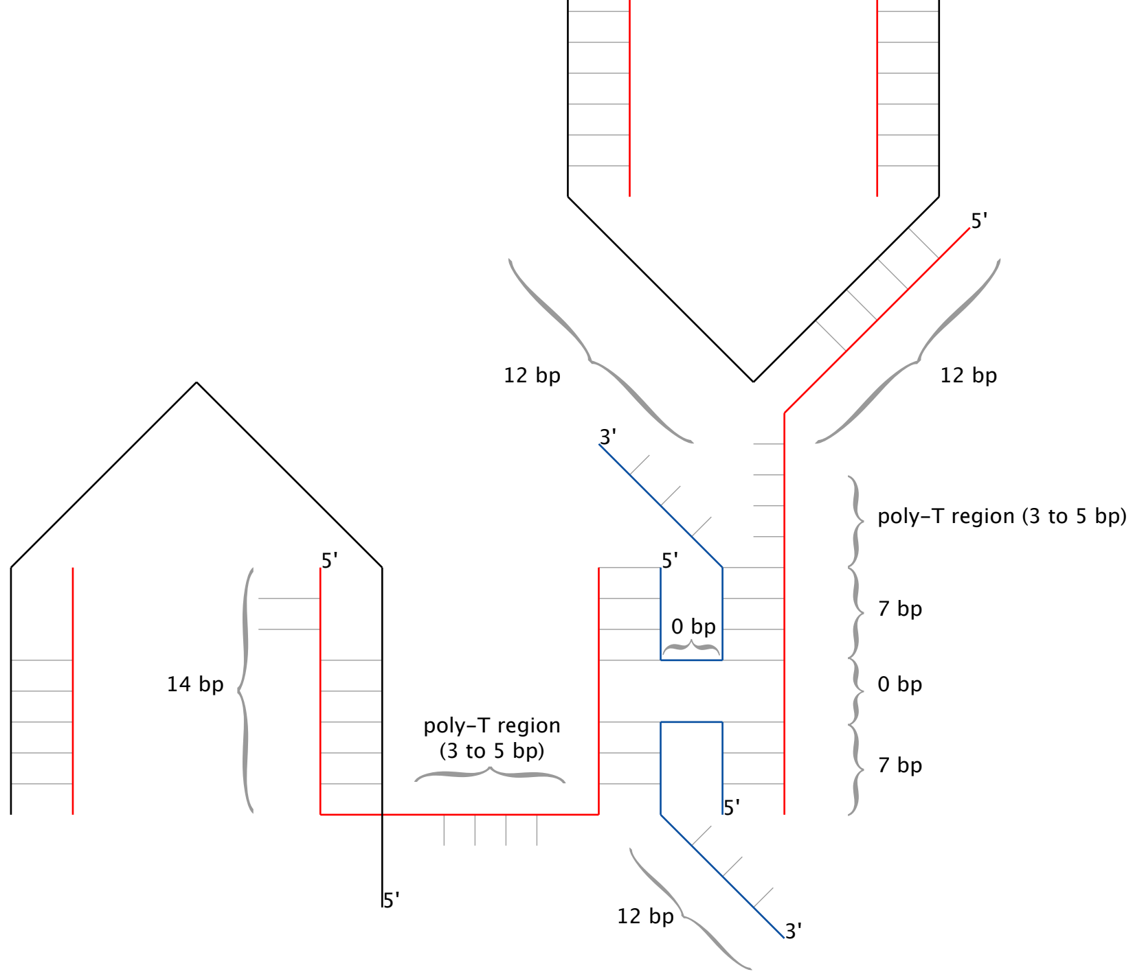
scaffold-oligo-staple-oligo-scaffold
