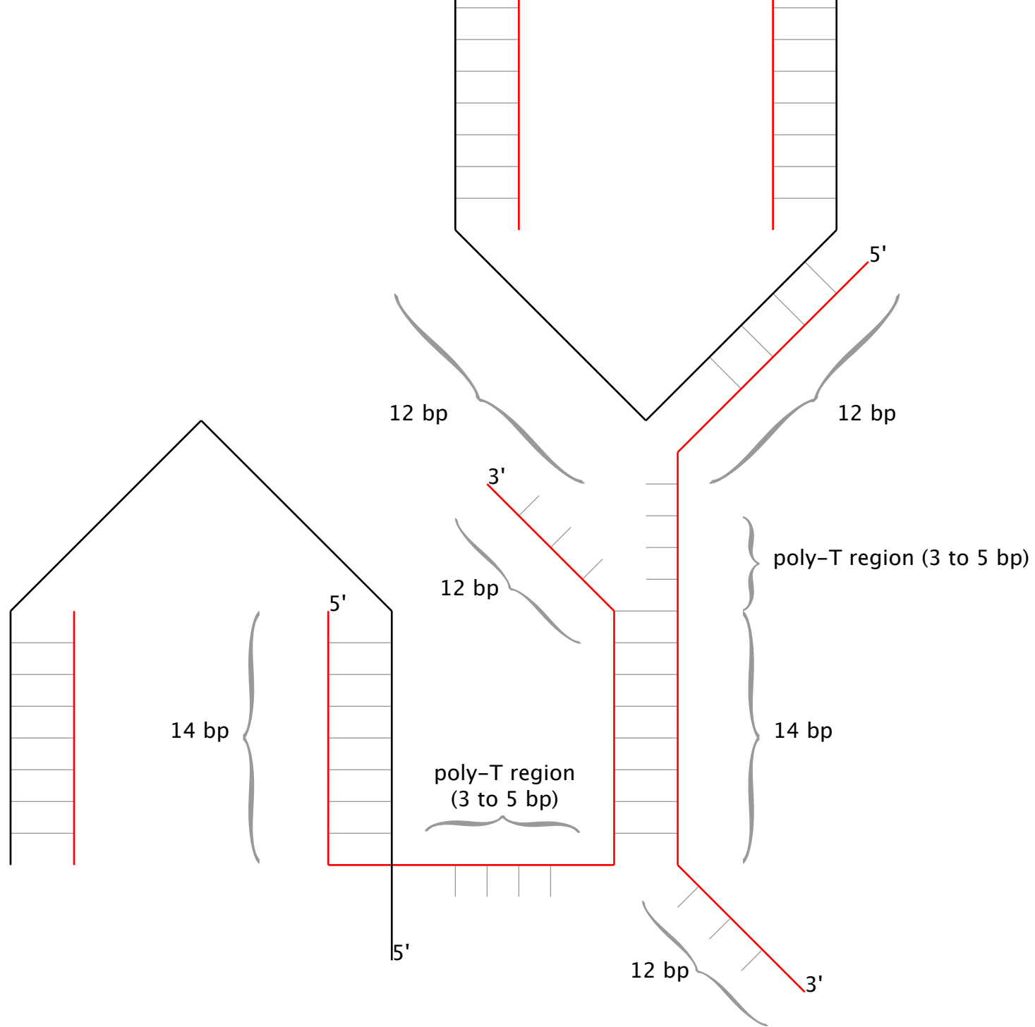
scaffold-oligo-oligo-scaffold
