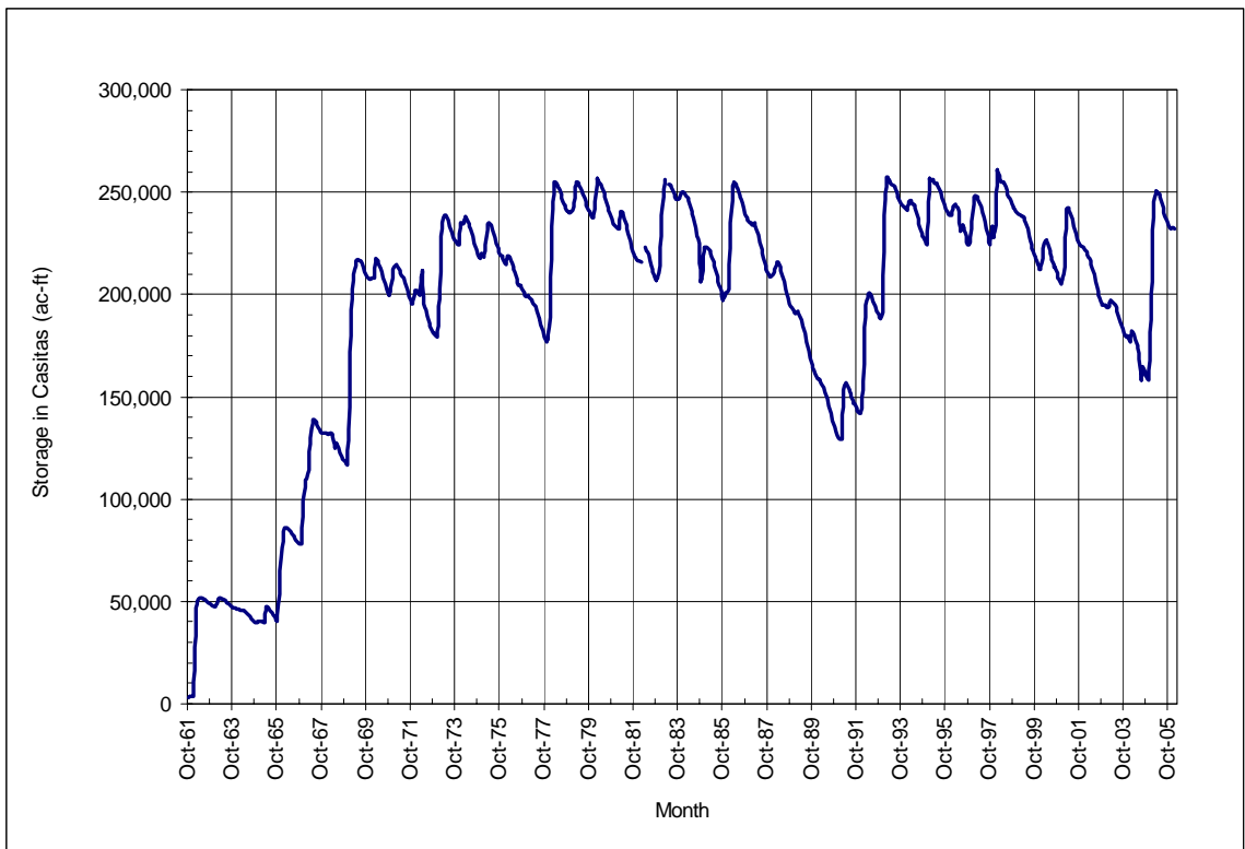
Figure 1.9. Storage in Lake Castitas.
